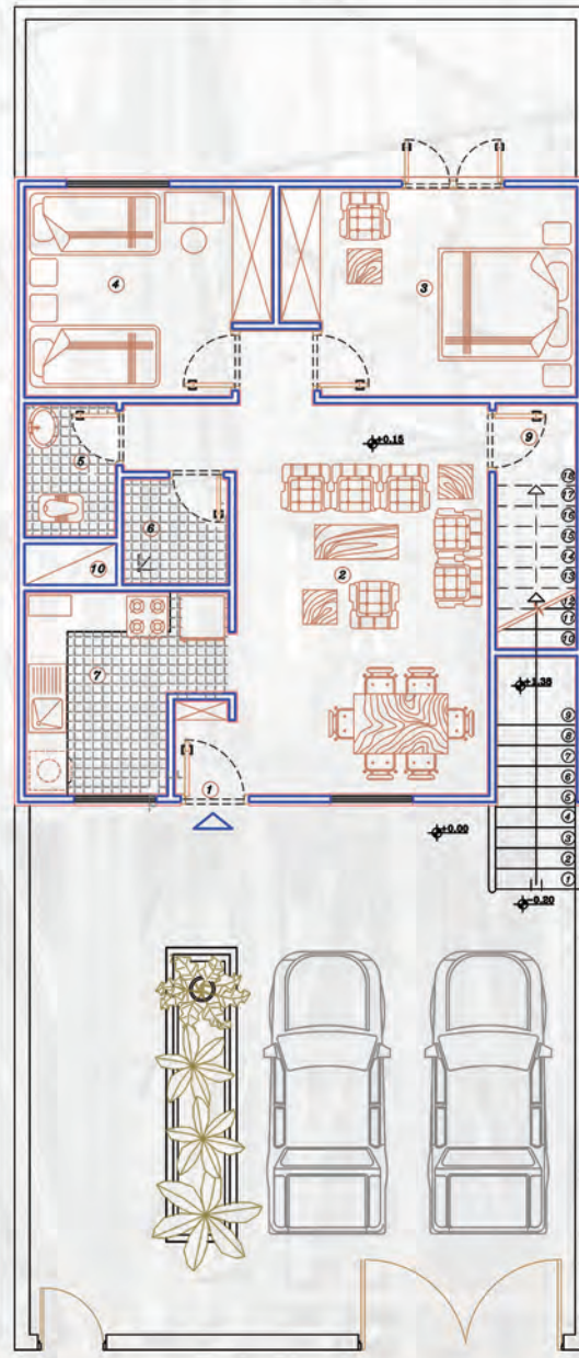
پلان طبقه همکف
